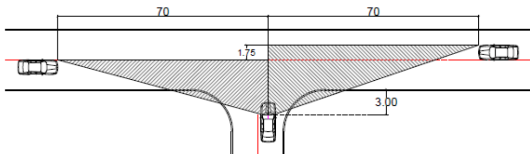
Redzamības brīvlauks šķērsojot veloceļu C, D kategorijas ceļam ar ātrumu V \leq 50 km/h
