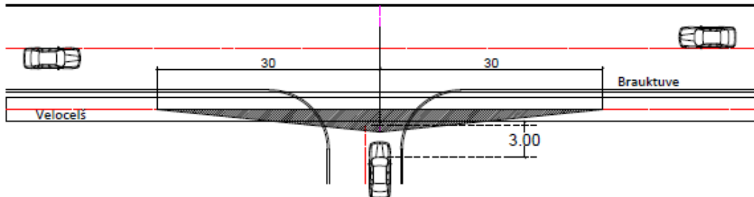
Redzamības brīvlauks E kategorijas ceļam ar ātrumu V \leq 20 km/h
