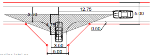
Redzamības brīvlauks D, E kategorijas ceļam ar ātrumu V \leq 30 km/h
