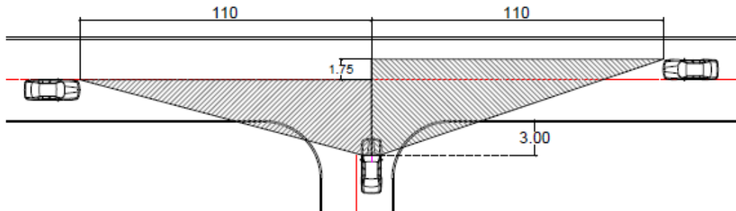
Redzamības brīvlauks B, C, D kategorijas ceļam ar ātrumu V \leq 50 km/h
