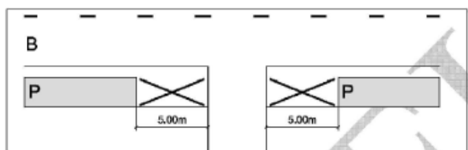
Autostāvvietu izvietojums C, D kategorijas ielai ar ātrumu V \leq 50 km/h
