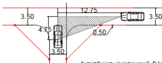
Autostāvvietu izvietojums C, D kategorijas ielai ar ātrumu V \leq 50 km/h
